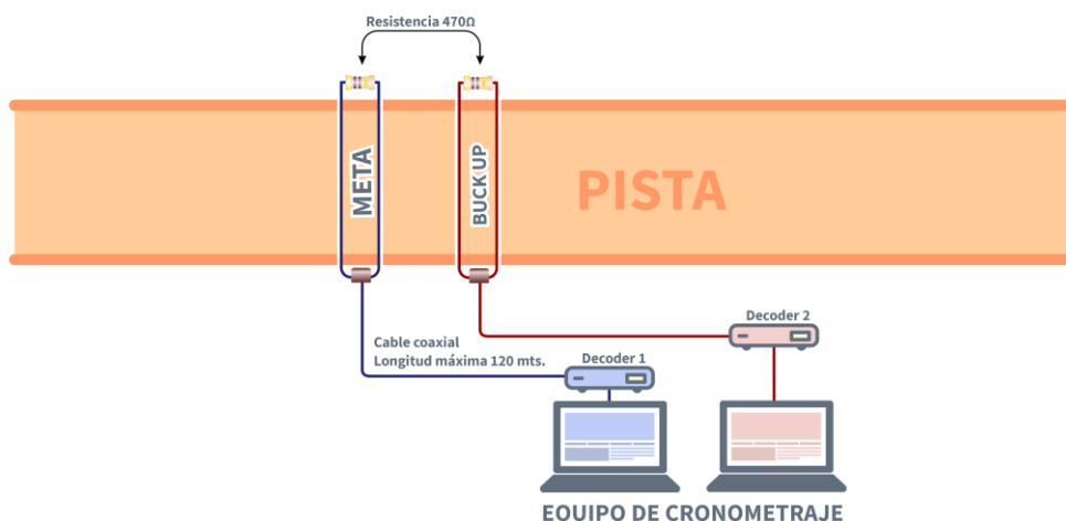
Esquema 1 (Instalación Global)
