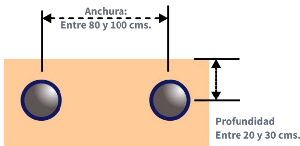
Esquema 2 (Instalación Antena/Bucle)
